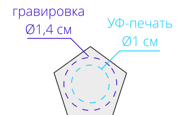
пятигранная панель
